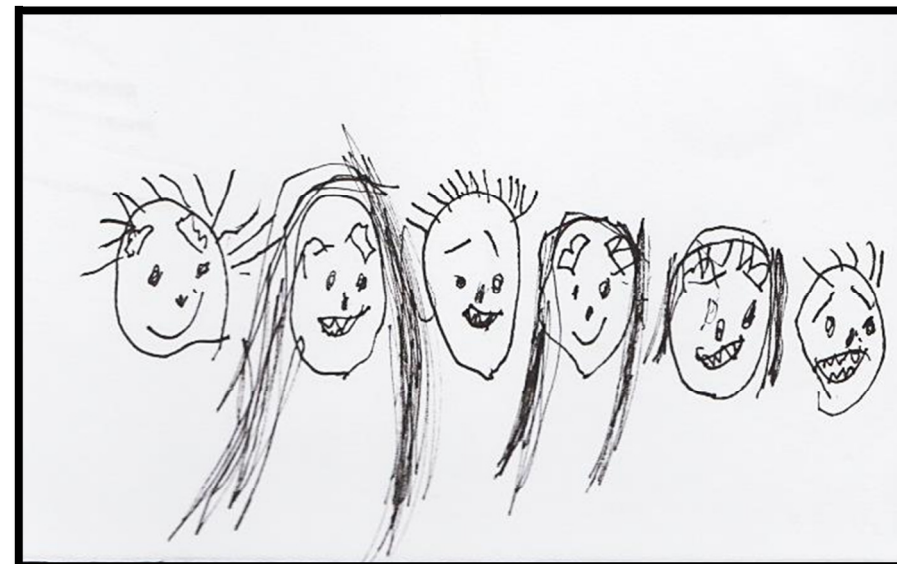
Två bakteriefamiljer
